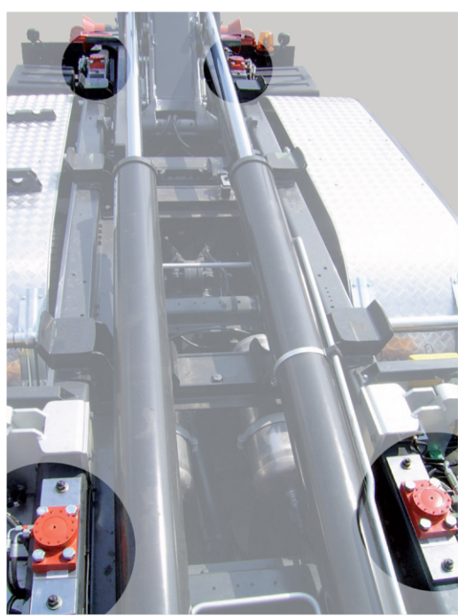
Группа WEIGHTPAD площадок на раме
