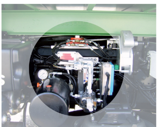
Соединительная коробка, распределитель и площадка
