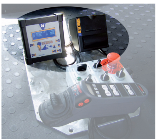
Индикатор и принтер в кабине
